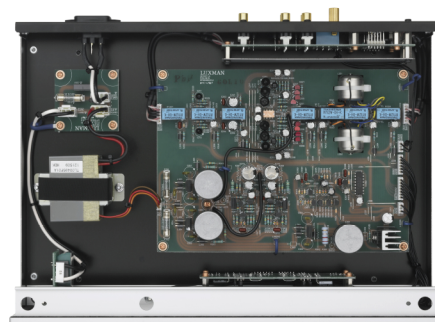
内部構成
