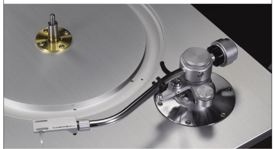
PD-171Aに標準装備のユニバーサル型トーンアーム
